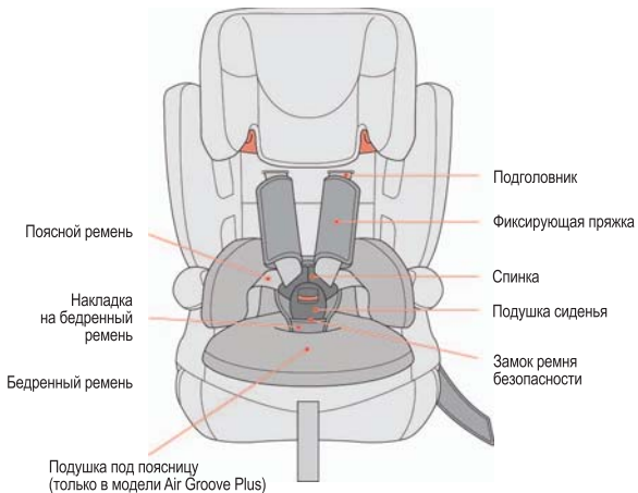
< Основной каркас: вид спереди >
