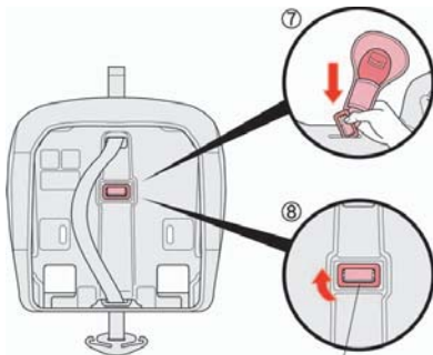
Конструкция внутри подушки сиденья
