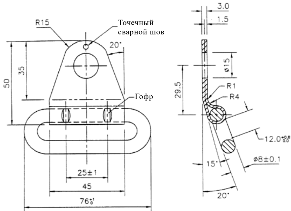
Рис. 4 Направляющая ремня безопасности Отделка: хромированное покрытие (Размеры в мм)
