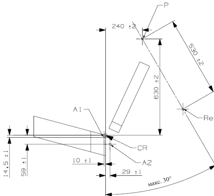
Вид сбоку – Стенд с креплениями ремня (общий допуск: \pm 2 мм)
